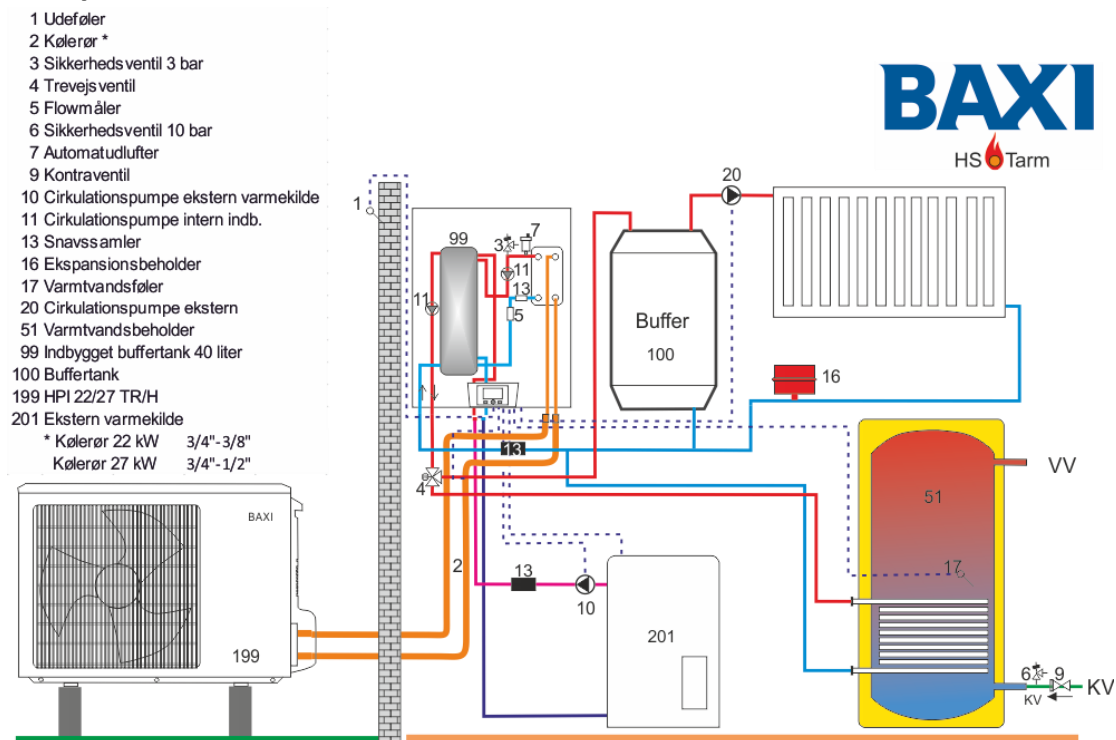
HPI 22/27 TR hybrid med 300 liter buffer, VVB og ekstern backup. ver.1
